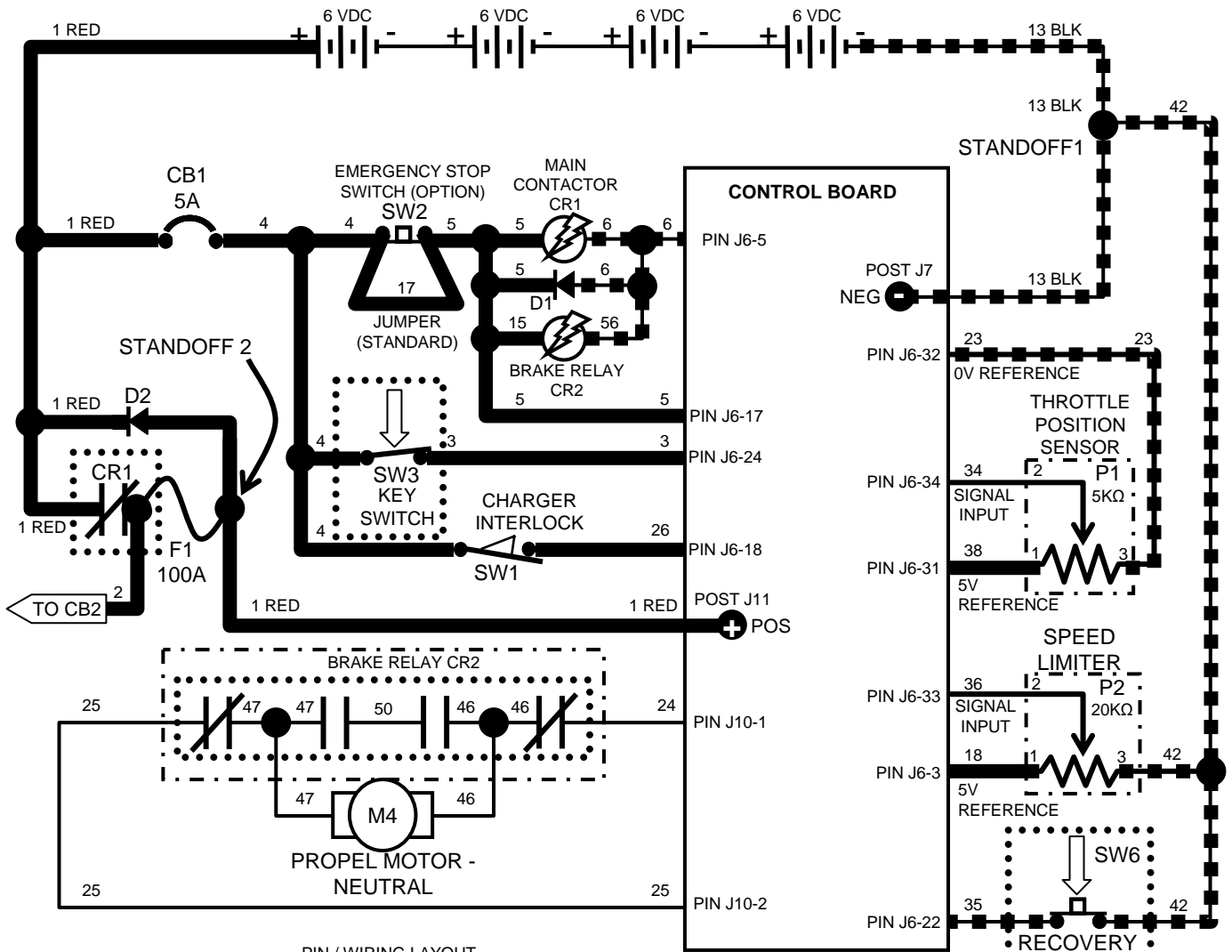
PIN / WIRING LAYOUT
